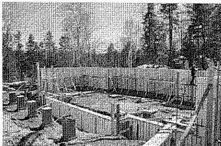
Coffrage isolant
